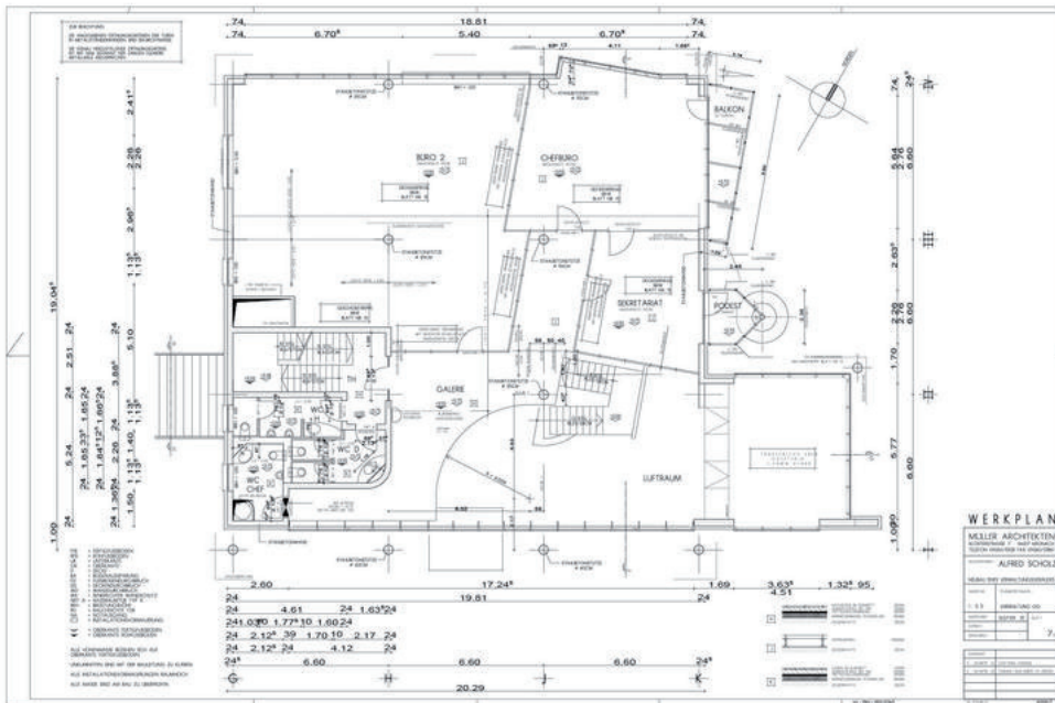
Grundriss des Obergeschosses (Bürogebäude)
